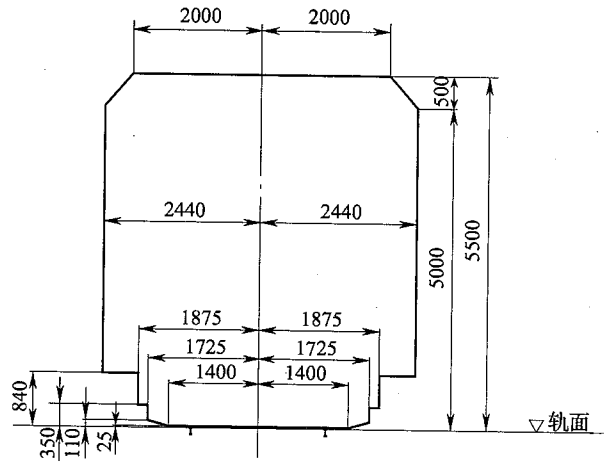
图 A. 2. 2 冶车线建筑限界(mm)
