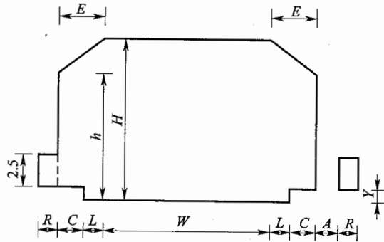
图 B.0.1 道路建筑限界
