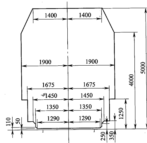
图 A.1.2 冶车车辆限界(mm)
