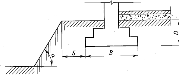
图 6.3.10 基础底面外边缘线至坡顶的水平距离
