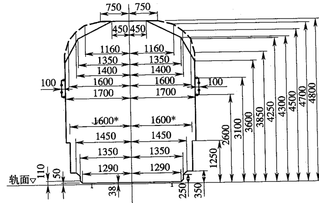
图 6 机车车辆上部限界 (mm)
