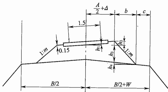
图 4 曲线地段路基加宽值
