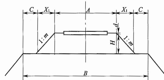
图 3 单线岩石、渗水土路基宽度
