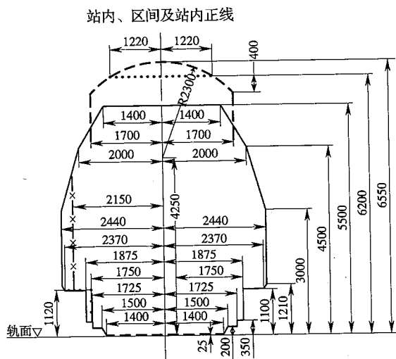
图7 基本建筑限界(mm)(建限-1)
