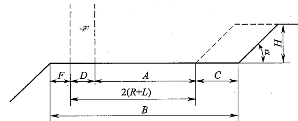
图5 排土场工作平台宽度
